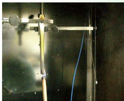
消火 Extinction
