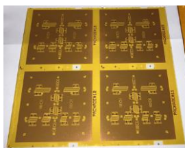
〈実機した基板の外観図〉
